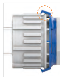
너트 체결 상태 불량 (과체결 상태) Nut拧紧状态不良 (过紧状态)
