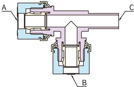
UNION TEE ADAPTOR (TUBE END)
