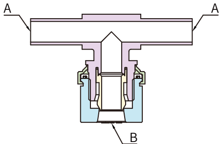
UNION TEE ADAPTOR (TUBE END)
