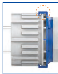
너트 체결 상태 양호 (조립 체결) Nut拧紧状态良好 (组装连接)
